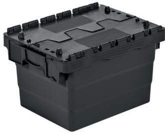
HP-4325-ESD En/W Boy/L Yüksek/H Dış / Ext 300 x 400 x 250 mm İç / Int 265 x 340 x 230 mm
