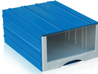
501-G En/W Boy/L Yük/H Dış / Ext 212 x 306 x 126 mm İç / Int 193 x 290 x 110 mm
