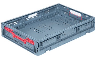
PG-6411 En/W Boy/L Yük/H Dış / Ext 400 x 600 x 115 mm İç / Int 376 x 576 x 106 mm Katlanmış Yükseklik 30 mm Folded Height 30 mm
