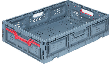
PG-6415 En/W Boy/L Yük/H Dış / Ext 400 x 600 x 150 mm İç / Int 376 x 576 x 141 mm Katlanmış Yükseklik 30 mm Folded Height 30 mm
