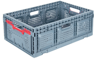
PG-6422 En/W Boy/L Yük/H Dış / Ext 400 x 600 x 219 mm İç / Int 362 x 576 x 210 mm Katlanmış Yükseklik 30 mm Folded Height 30 mm
