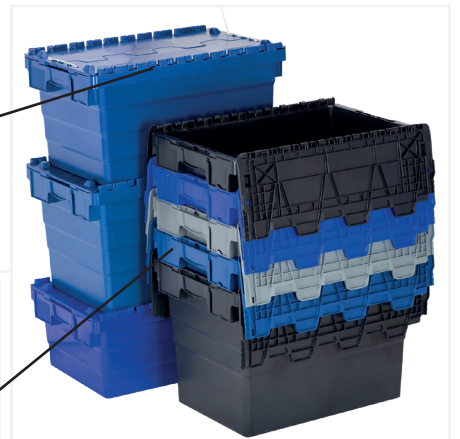
HP-4336-ESD En/W Boy/L Yüksek/H Dış / Ext 300 x 400 x 365 mm İç / Int 265 x 340 x 345 mm
