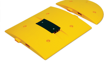
12112 YK En/W Boy/L Yüksek/H 500 x 500 x 45 mm Ağırlık / Weight 3,10 Kg Material : PPC
