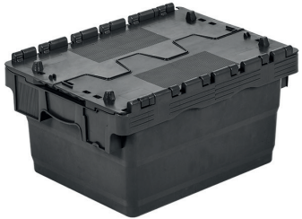
HP-4321-ESD En/W Boy/L Yüksek/H Dış / Ext 300 x 400 x 210 mm İç / Int 265 x 340 x 190 mm
