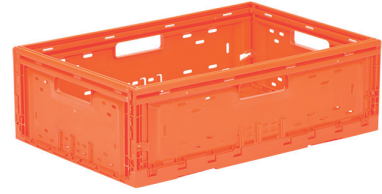
KT-6420 En/W Boy/L Yük/H Dış / Ext 400 x 600 x 197 mm İç / Int 372 x 573 x 193 mm Katlanmış Yükseklik 32 mm Folded Height 32 mm
