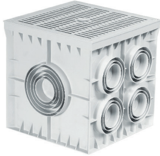
LOGA 056 En/W Boy/L Yükseklik / H 550 x 550 x 500 mm Çıkış Adedi / Connections : 10 Ad / Pcs
