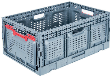
PG-6426 En/W Boy/L Yük/H Dış / Ext 400 x 600 x 259 mm İç / Int 376 x 576 x 251 mm Katlanmış Yükseklik 47 mm Folded Height 47 mm
