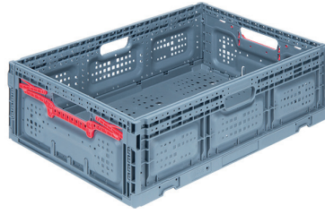
PG-6418 En/W Boy/L Yük/H Dış / Ext 400 x 600 x 185 mm İç / Int 362 x 576 x 176 mm Katlanmış Yükseklik 30 mm Folded Height 30 mm
