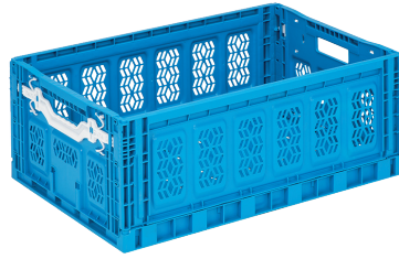
KTA-6422 En/W Boy/L Yük/H Dış / Ext 400 x 600 x 225 mm İç / Int 372 x 572 x 215 mm Katlanmış Yükseklik 40 mm Folded Height 40 mm
