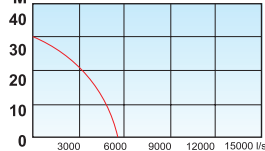
YÜKSEKLİK DEBİ GRAFİĞİ
