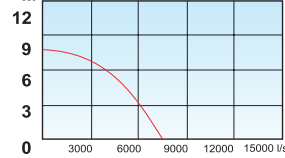
YÜKSEKLİK DEBİ GRAFİĞİ
